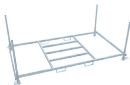
Horizontaal transport
